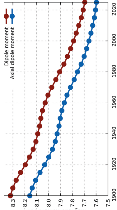
Velikost Zemljinega dipolnega magnetnega momenta od leta 1900 do leta 2020
