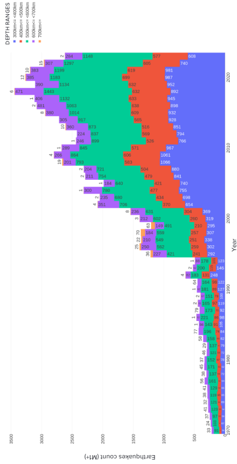
Potresi z globokim žariščem M1+ po svetu v obdobju 1970–2023
