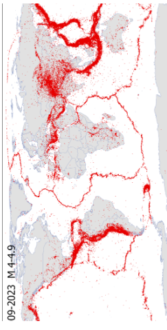
Potresi M4,0–4,9 po svetu v obdobju 2009–2023
