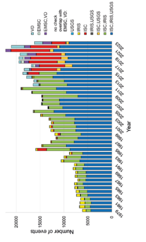
Število edinstvenih potresov M4+ v obdobju 1979–2023, o katerih so poročale samo navedene službe
