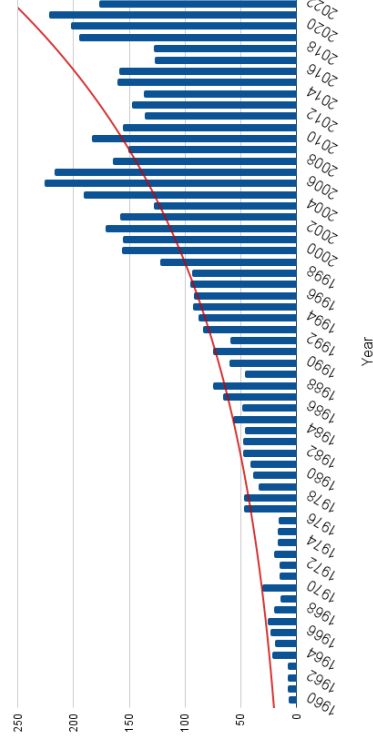
Skupno število poplav velikega obsega na svetu
