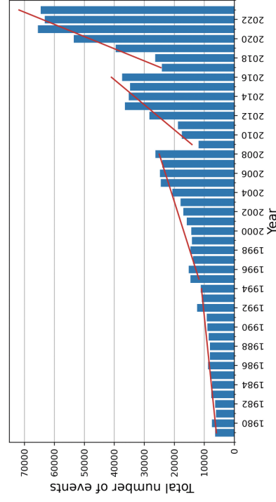
Potresi M3–M9 po svetu v obdobju 1979–2023
