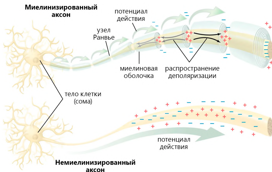
Рисунок 83. Нейрон: проведение потенциала действия.
