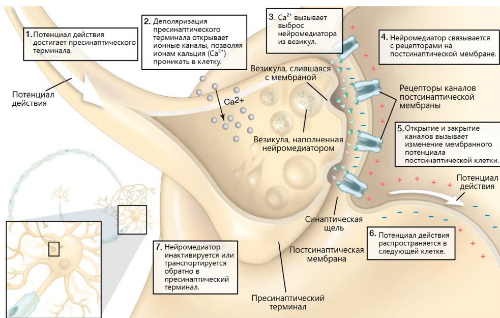
Рисунок 82. Синапс Химическая передача нервного импульса в синапсе. Поступление нервного импульса в пресинаптическое окончание стимулирует высвобождение нейромедиаторов в синаптическую щель. Связывание нейромедиаторов с рецепторами на постсинаптической мембране стимулирует регенерацию потенциала действия в постсинаптическом нейроне.
