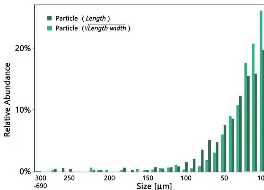
Рисунок 61. Относительное распределение частиц микропластика по размерам для всех проанализированных станций ( n = 543 ). На изображениях показаны самые маленькие (справа) и самые большие (слева) частицы МР, обнаруженные и подтвержденные с помощью Раман-микроспектрометрии.
