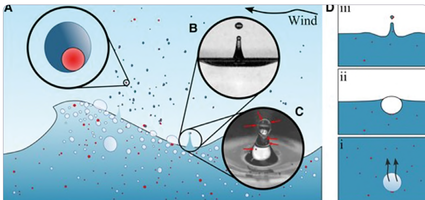
Рисунок 13. Рисунок соответствующих процессов выброса микропластика из океана. А) Микропластик (красный / более тёмный цвет) в океане переносится в атмосферу каплями морской воды. В) Лопающиеся пузырьки создают небольшие капли или аэрозоли, такие как струйные капли. С) Микропластик, присутствующий в жидкости, может переноситься в образующиеся струйные капли. Стрелки указывают на микропластиковые частицы размером 100 \mu\text{m} . Образующиеся капли могут подхватываться ветром и переносить микропластиковый материал в атмосферу. Жидкость в конечном итоге испаряется, оставляя микропластиковые частицы. D) Соответствующие физические процессы выброса микропластика путём лопания пузырька начинаются с очистки частиц по мере подъёма пузырька Di). После достижения поверхности Dii) пузырёк в конечном итоге принимает свою равновесную форму, которая после лопания фокусирует капиллярные волны у своего основания, образуя струйные капли Diii), переносящие микропластиковый материал.
