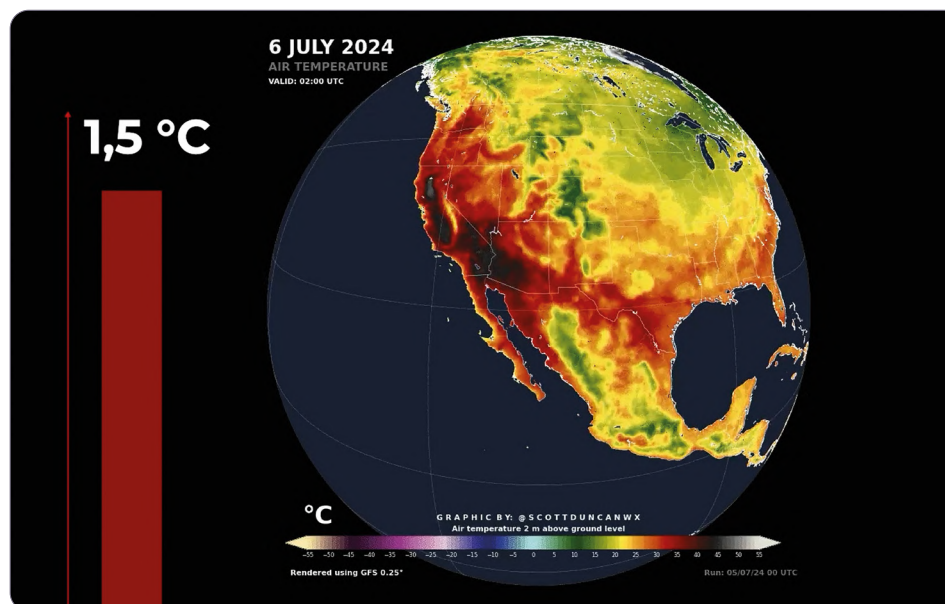
Рисунок 44. Схематическое отображение климатического рубежа: в 2024 г. среднегодовая глобальная температура впервые превысила порог в 1,5 °C по сравнению с доиндустриальным уровнем
