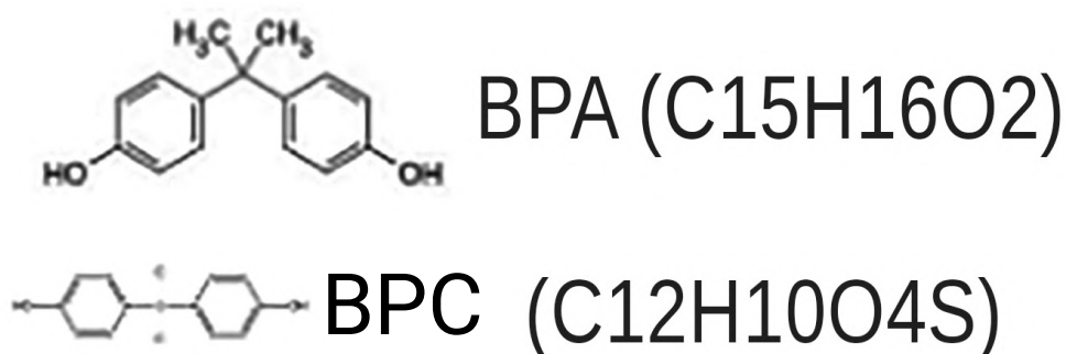
Рисунок 76. Молекулярные структуры и химические формулы бисфенола А (BPA) и бисфенола-С (BPC).
