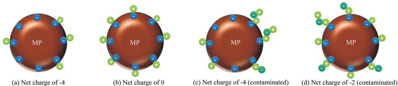
Рисунок 101. Иллюстрация эффекта поверхностных зарядов микропластика, вызванных загрязняющими веществами воды.
