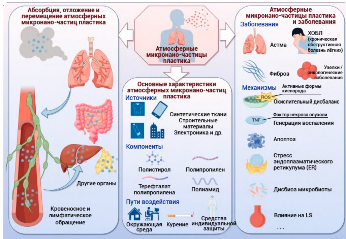
Рисунок 86. МНП: источники, пути попадания и токсические эффекты.
