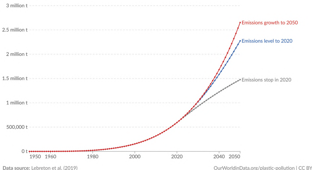
Рисунок 29. График роста количества микропластика на поверхности океана с прогнозом до 2050 года. https://ourworldindata.org/grapher/microplastics-in-ocean (Дата доступа 01.05.2025)
