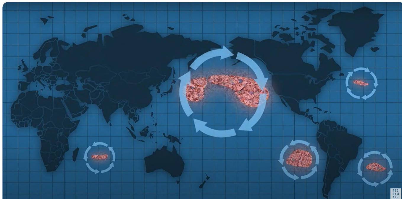
Рисунок 5. Схематическое изображение пяти крупных скоплений мусора в Мировом океане: два — в Атлантическом океане, два — в Тихом океане и одно — в Индийском океане. В океанах циркулируют миллионы тонн пластика и других отходов антропогенного происхождения. Мусорные пятна растут в катастрофической прогрессии.
