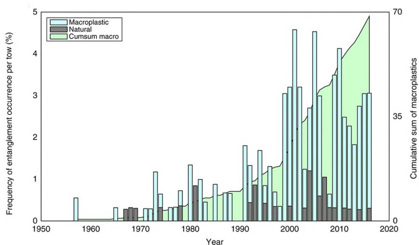
Рисунок 97. Рост количества пластика в океане с 1957 по 2020 гг.
