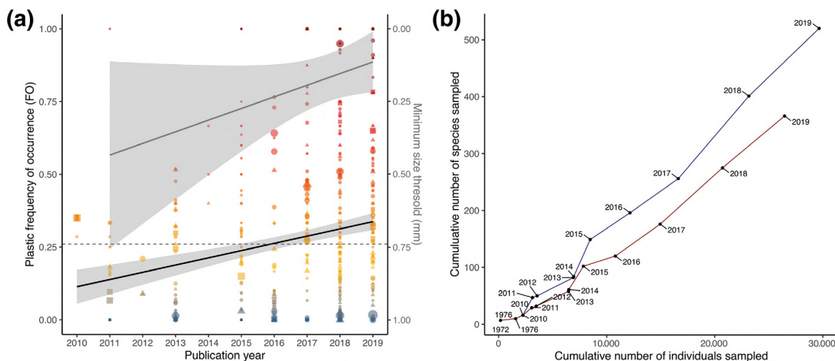
Рисунок 30. Временные тенденции потребления пластика рыбами. (а) Верхняя серая линия указывает на то, что с 2011 года наблюдается тенденция к обнаружению всё более мелких частиц. Нижняя чёрная линия показывает увеличение частоты встречаемости пластика (FO) среди всех видов рыб с 2010 по 2019 год. В течение этого периода частота потребления пластика значительно возросла со скоростью 2,4 % в год. Горизонтальная пунктирная линия представляет FO 0,26, среднюю частоту потребления пластика рыбами во всём мире. (б) Кривая накопления видов, где синяя линия указывает на совокупное количество видов, изученных с течением времени, включая виды, обнаруженные с поглощённым пластиком и без него, а красная линия изображает только виды с поглощением пластика. Отсутствие асимптоты на красной линии указывает на высокую вероятность того, что в ближайшие годы будут продолжаться появляться дополнительные виды, которые будут поглощать пластик. Savoca, M. S., McInturf, A. G. & Hazen, E. L. Plastic ingestion by marine fish is widespread and increasing. Global Change Biology 27, 2188–2199 (2021). https://doi.org/10.1111/gcb.15533
