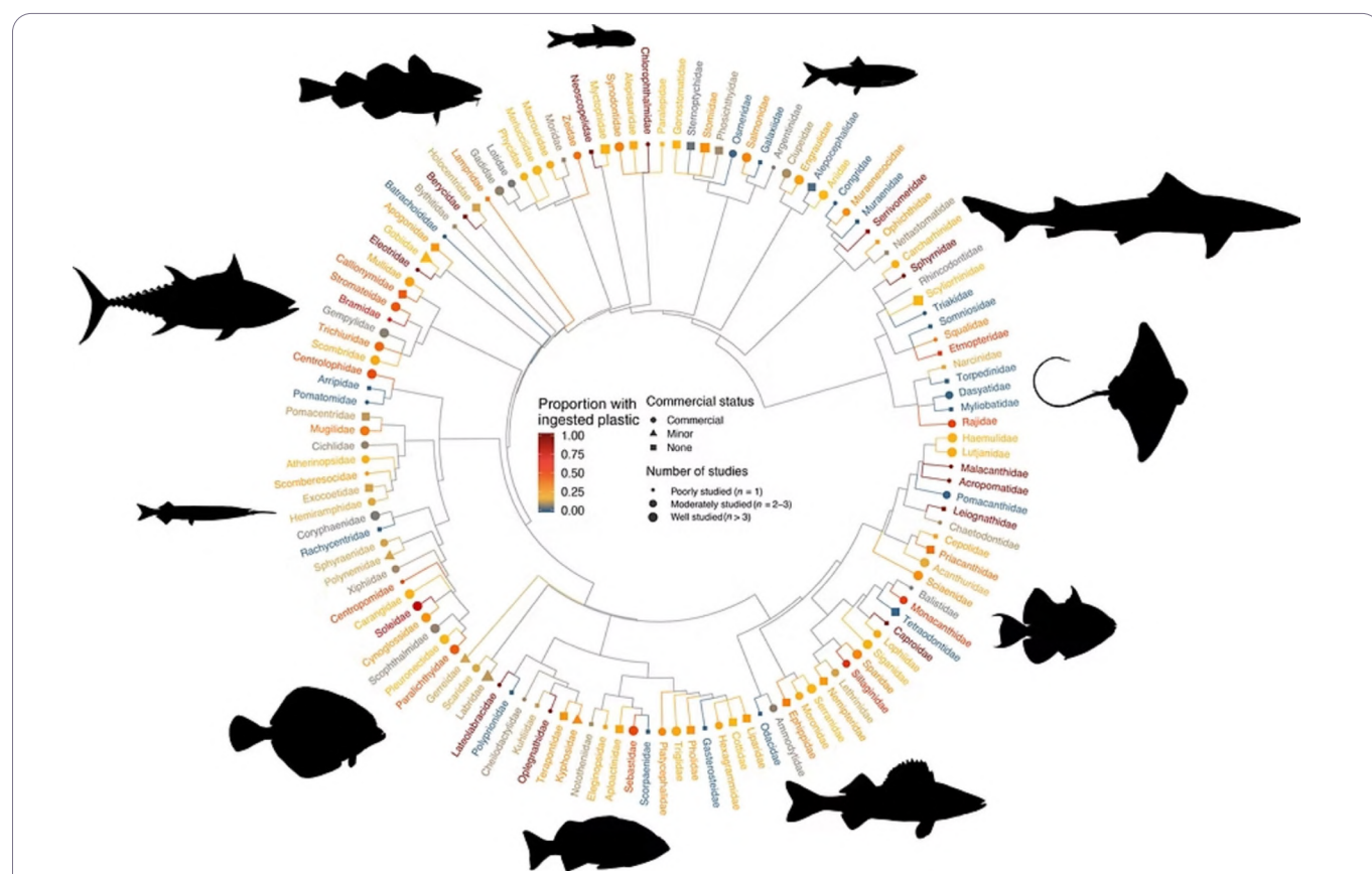
Рисунок 28. Семейства рыб и проглатывание пластика
