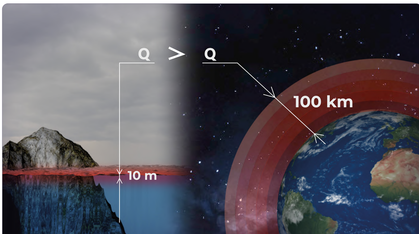
Рисунок 38. Сравнительная теплоёмкость океана и атмосферы: несмотря на меньшую массу воздуха, океан способен накапливать и удерживать в десятки раз больше тепла, играя ключевую роль в регулировании климата Земли
