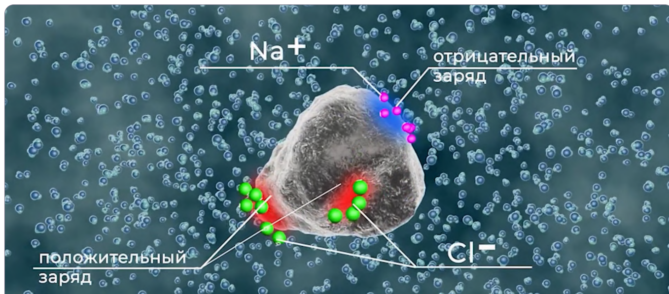
Рисунок 58. Схематическое изображение процесса формирования гидратной оболочки вокруг заряженных наночастиц пластика: в данном процессе наночастицы, обладая зарядом, притягивают ионы, что способствует образованию вокруг них молекул воды, создавая защитную гидратную оболочку.
